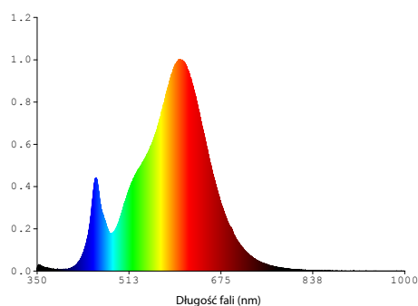
LEDSTAR ECO GU10, 7W, CB - 3000K
